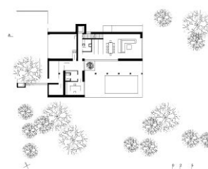
Grundriss Obergeschoß
